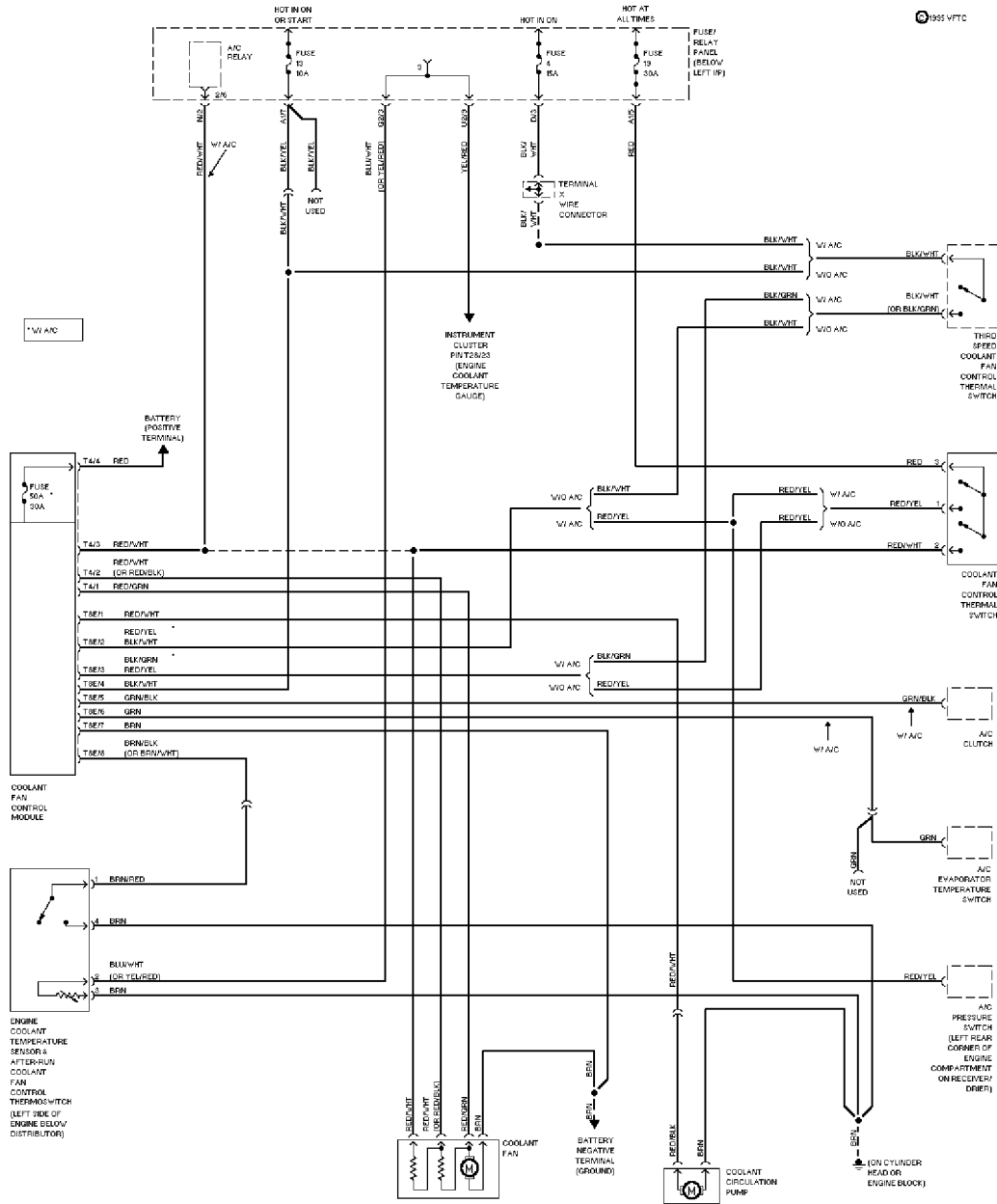
1994 Cooling Fan Circuit
