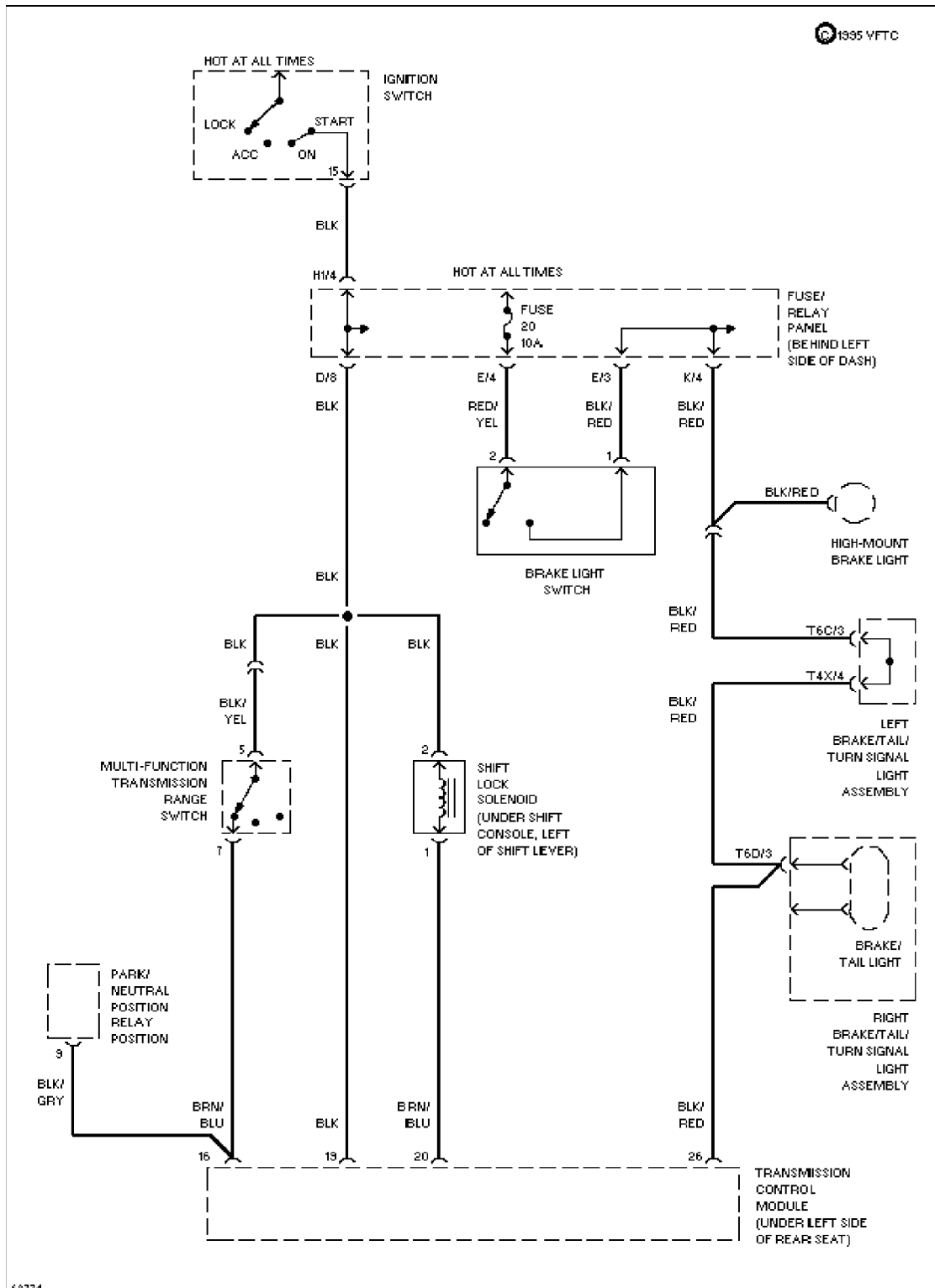
68774 Shift Interlock Circuit
